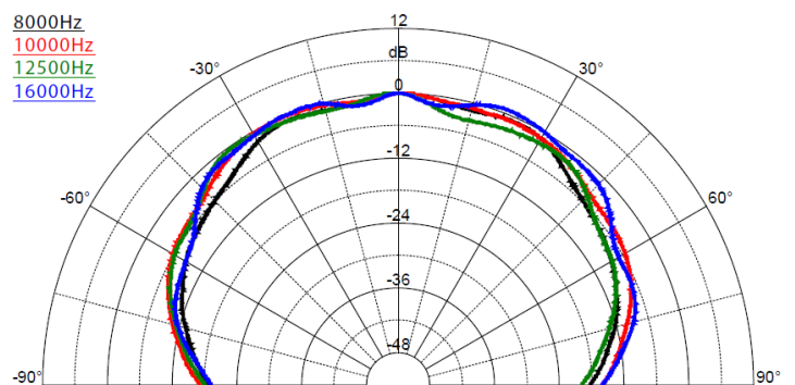
SAROS IC8T – Диаграмма направленности, 8000 Гц – 16000 Гц
