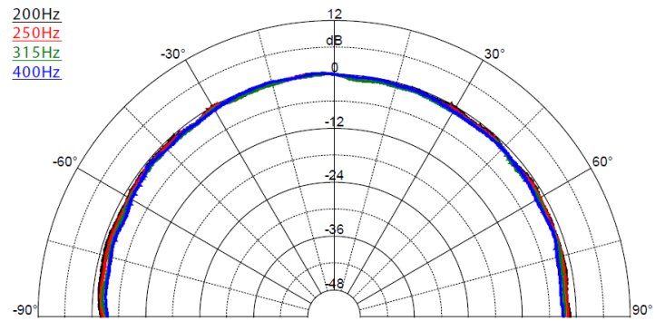
SAROS IC4T – Диаграмма направленности, 200 Гц – 400 Гц
