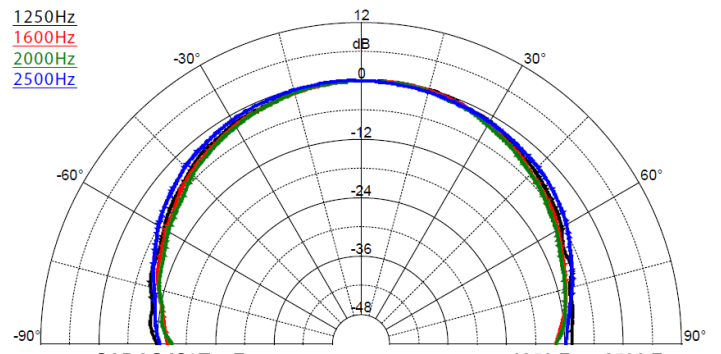
SAROS IC8T – Диаграмма направленности, 1250 Гц – 2500 Гц
