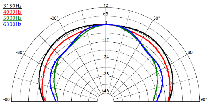
SAROS IC4T – Диаграмма направленности, 3150 Гц – 6300 Гц
