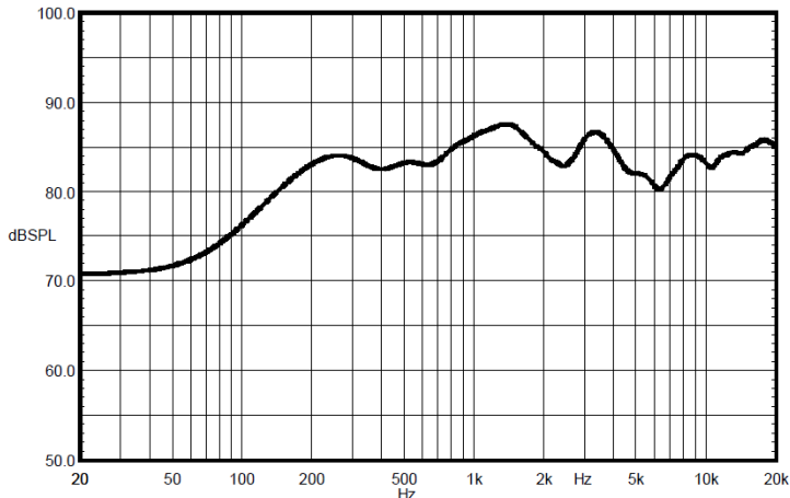
SAROS IC4T – Частотная характеристика
