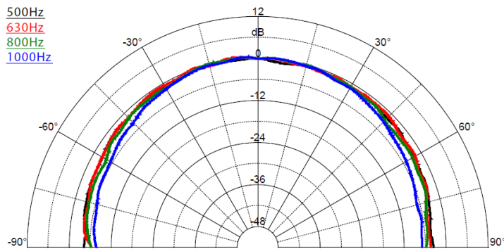
SAROS IC4T – Диаграмма направленности, 500 Гц – 1000 Гц
