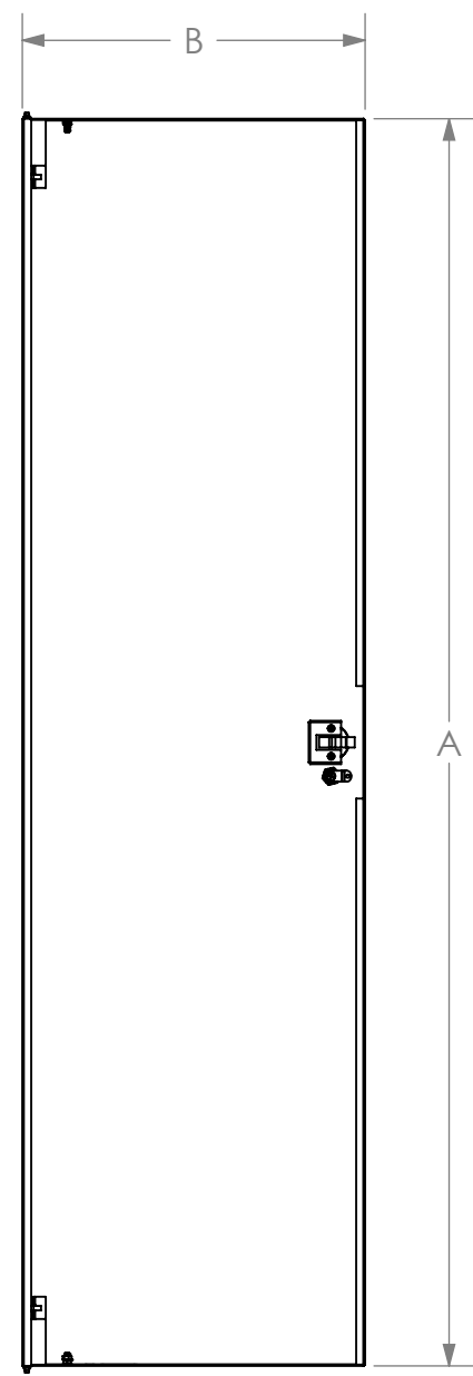
SOLID DOOR
