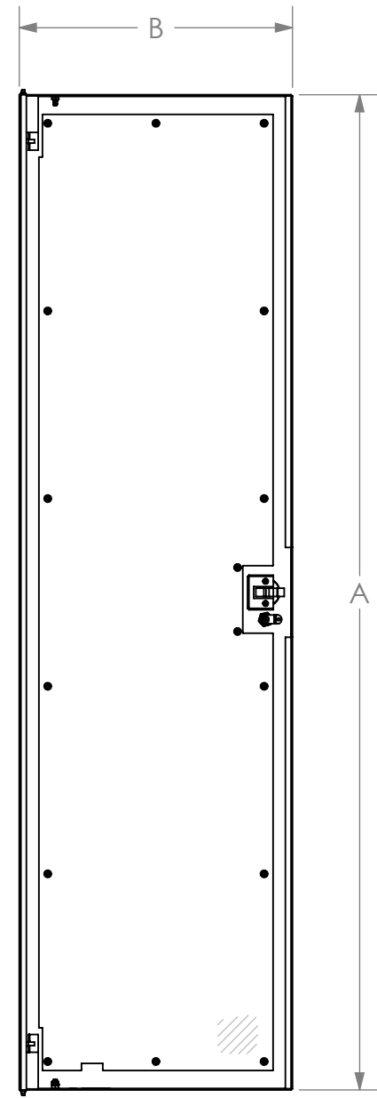
PLEXIGLASS DOOR
